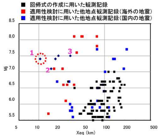
図5. 関西電力が第59回新規規制基準適合性に係る審査会合(2013.12.18)で示した耐専スペクトルの適用性検討データ(1:FO-A~FO-B断層(M7.4, Xeq=10.5km), 2:熊川断層(M7.1, Xeq=15.4km), 3:上林川断層(M7.5, Xeq=30.2km))
