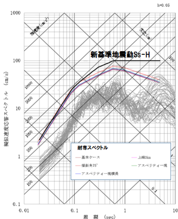
図 8: 高浜原発における FO-A~FO-B 断層と熊川断層の連動を考慮した場合の耐専スペクトルと断層モデルによる地震動評価結果 (全ケース : NS 方向) および新基準地震動 Ss-H (水平方向) (2013 年 12 月)[21, 23]
