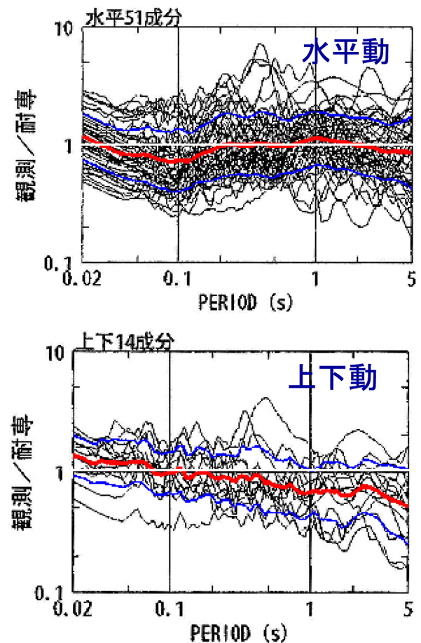
図 27: 国内外の内陸地殻内地震による震源近傍の観測記録 (M6.0~8.1, X_{eq} = 6 \sim 33 km, 水平 51 記録, 上下 14 記録) の耐専スペクトル (内陸補正有) との残差 (バラツキ)[34] (細線: 各地震観測記録に対する残渣, 太い赤実線: 残渣の平均, やや太い青実線: 平均からの「倍半分」の差)
