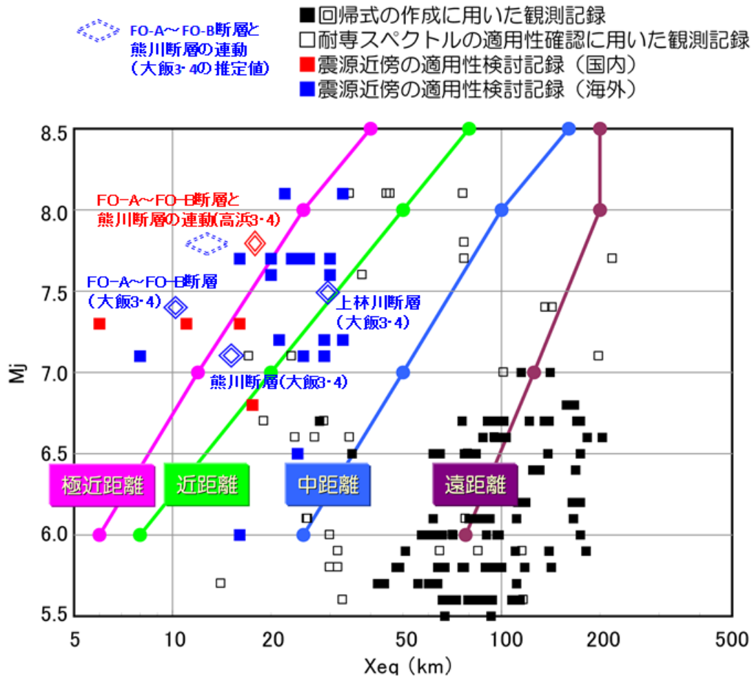
図 21: 耐専スペクトルの作成・適用性確認に用いられた地震データの等価震源距離 X_{eq} と気象庁マグニチュード M (図中では M_j と表記) [34] (大飯 3.4 号と高浜 3.4 号に関するデータを二重線の菱形 [22, 23] および二重点線の菱形 (推定値) で加筆した)
