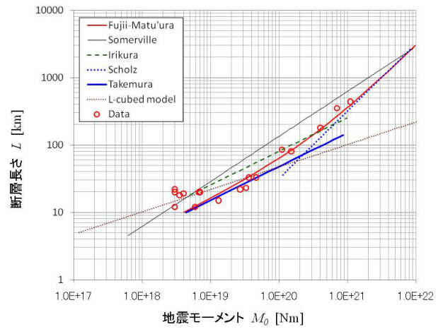
図 18: Fujii-Matsu'ura[5] 等によるスケールン則の関係：Somerville(細線)，入倉 (Irikura, 緑破線)，Scholz(青太点線)，武村 Takemura(青太直線)，L3 乗モデル (茶細点線)，Fujii-Matsu'ura(赤太曲線)．Fujii-Matsu'ura は Takemura と Scholz に漸近し国内地震データ (赤丸) にフィットしている
