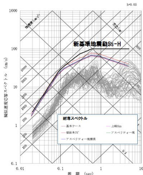
図1. 高浜原発におけるFO-A～FO-B断層と熊川断層の連動を考慮した場合の耐専スペクトル(折れ線)と断層モデルによる地震動評価結果(波線の重なり、全ケース：EW方向)および新基準地震動Ss=H(水平)(2013年12月)
