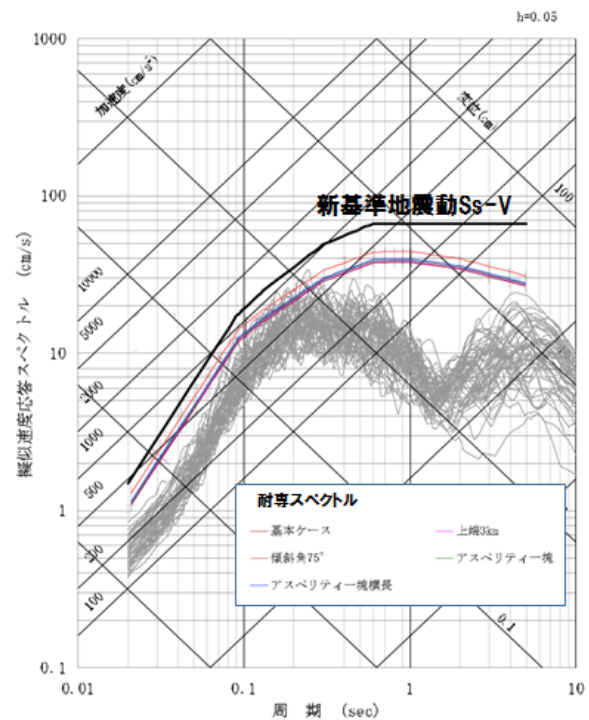
図 10: 高浜原発における FO-A~FO-B 断層と熊川断層の連動を考慮した場合の耐専スペクトルと断層モデルによる地震動評価結果 (全ケース : UD 方向) および新基準地震動 Ss-V (鉛直方向) (2013 年 12 月)[21, 23]
