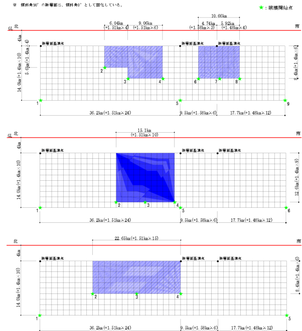
図 7: 高浜原発における FO-A~FO-B 断層と熊川断層の連動を考慮した断層モデル（上 2 つが「基本ケース」、下 2 つが不確実さを考慮した「アスペリティーが塊のケース」と「横長のケース」）[23]
