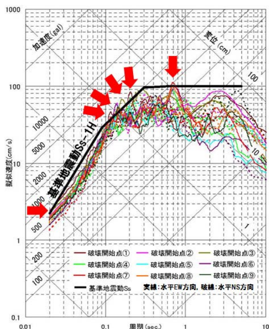
図2. 大飯原発におけるFO-A～FO-B断層と熊川断層の連動を考慮した場合の断層モデルによる地震動評価結果(応力降下量1.5倍ケース)と基準地震動Ss=1H(断層モデルでも6カ所で基準地震動を超えている：2013.12)
