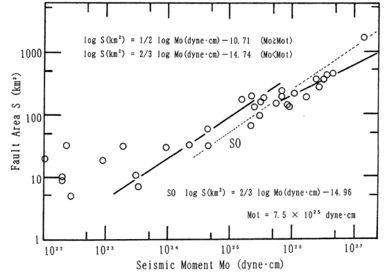
図 16: 武村 [32] による S - M_0 の関係
